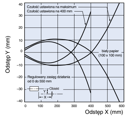
Modele odbiciowe od obiektu (osiowe) E3F2-DS30□4□
