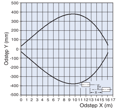
Modele odbiciowe z reflektorem (osiowe) E3F2-R2R□4□ (z polaryzacją) oraz reflektory
