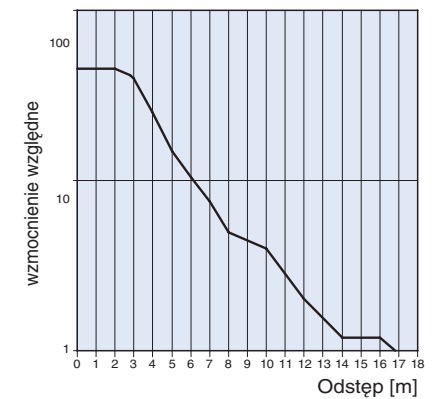
Modele typu nadajnik-odbiornik (osiowe) E3F2-10□
