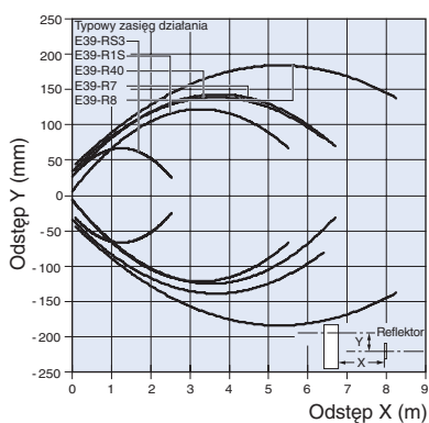
Modele odbiciowe z reflektorem (osiowe) E3F2-R4□4□ (z polaryzacją)
